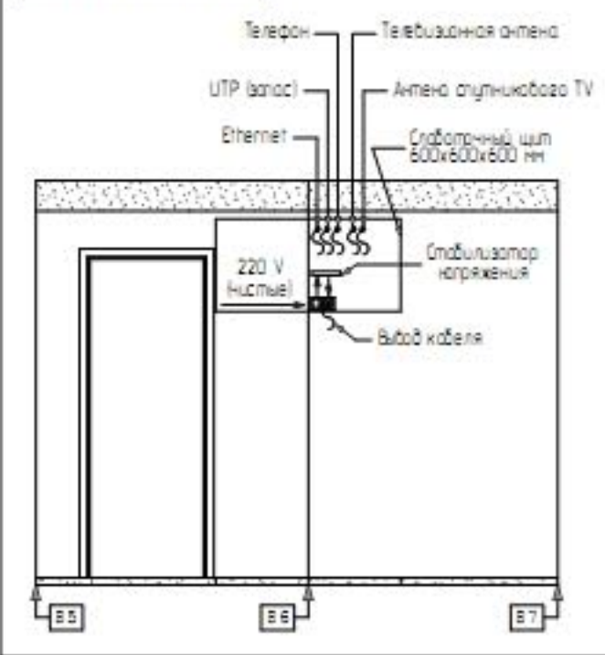
Принципиальная схема устройства слаботочного щита
